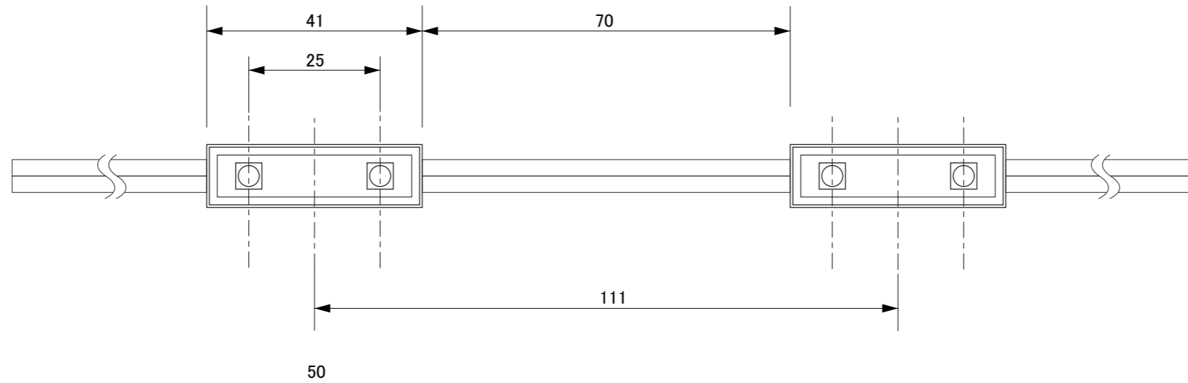
【上面図】
