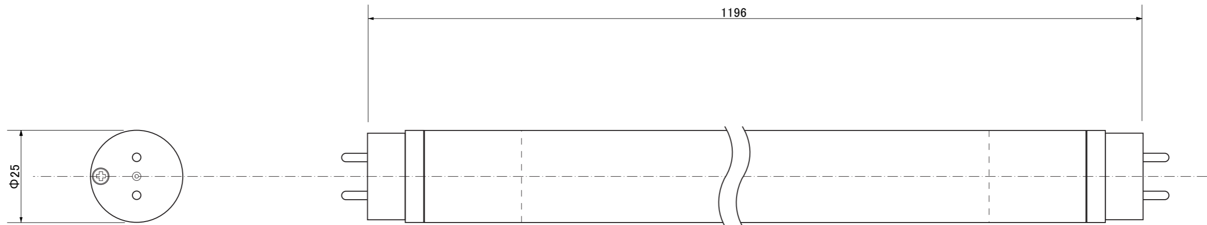
【上面図】
