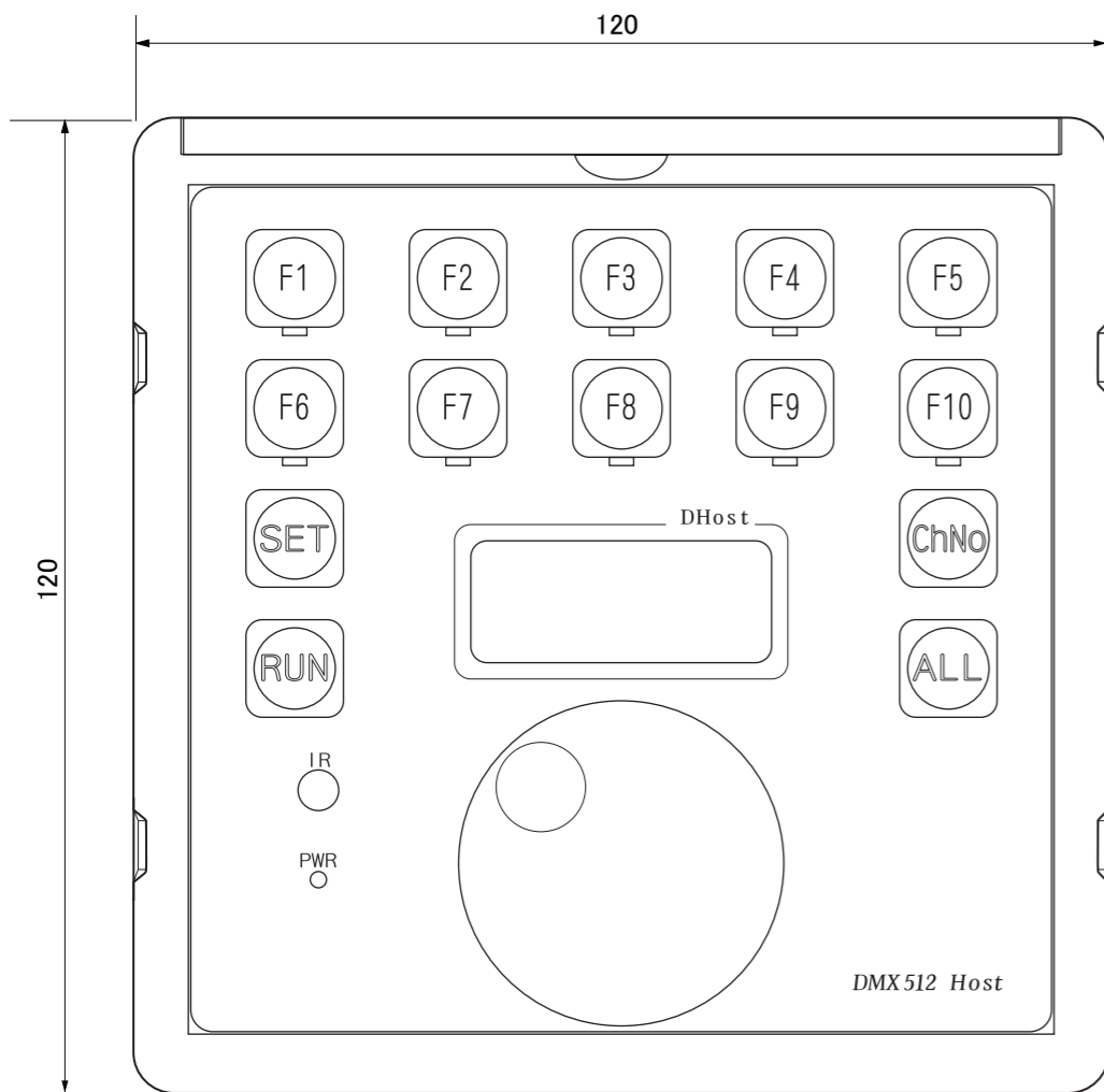
【正面図】
