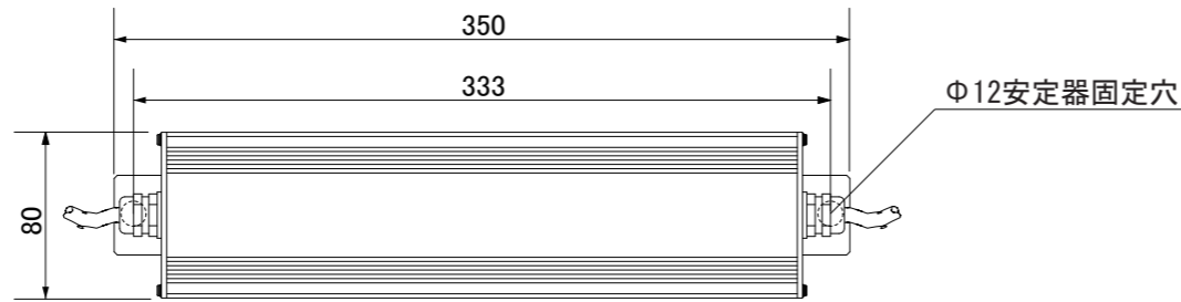
【上面図】
