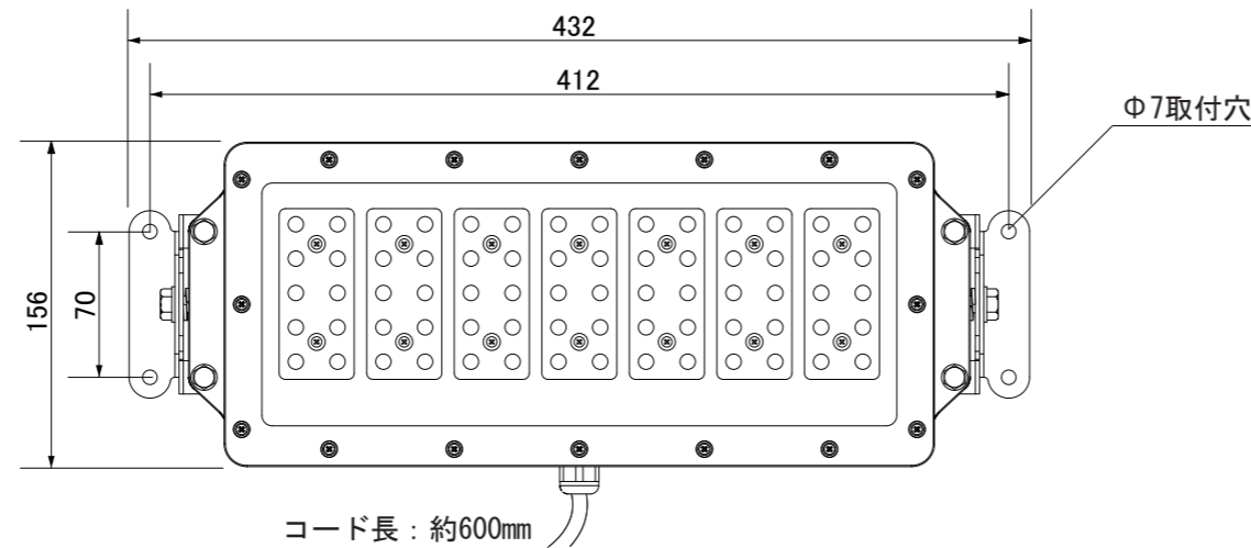
【正面図】
