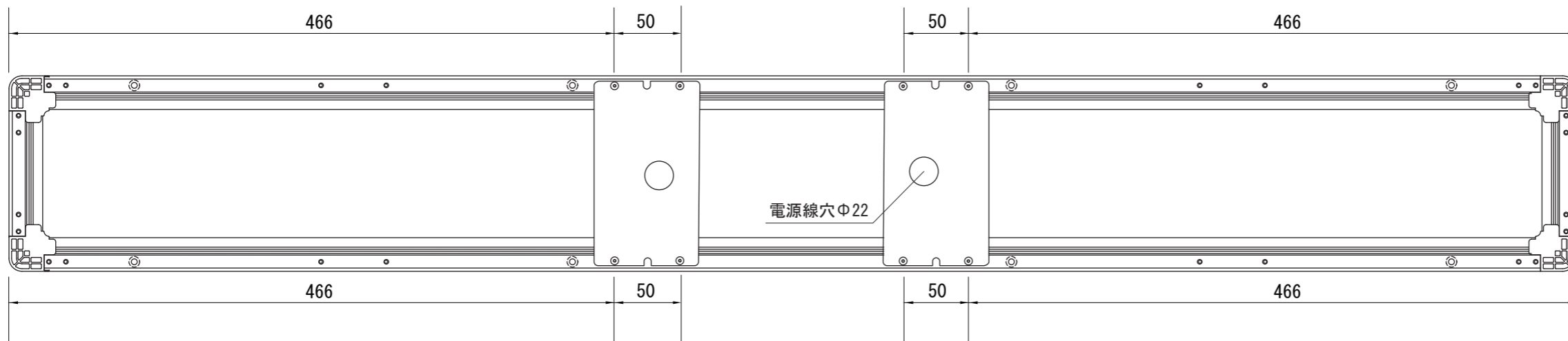
【背面図】
