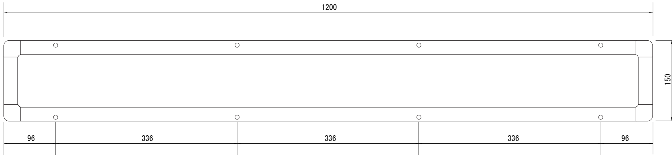
【正面図】
