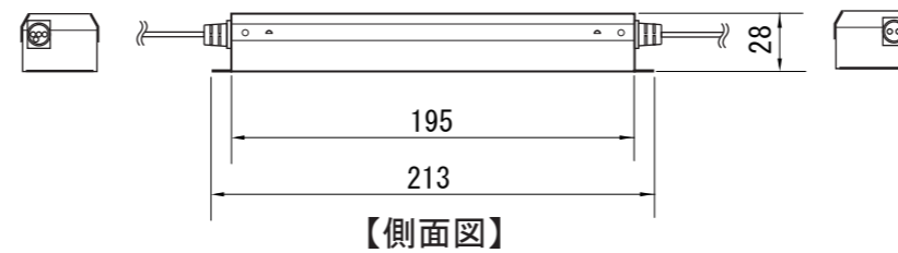
【正面図】
