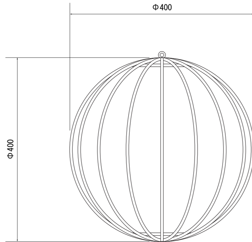
【正面図】
