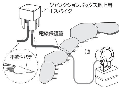
地中配線する場合
