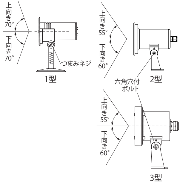
灯部可動範囲
