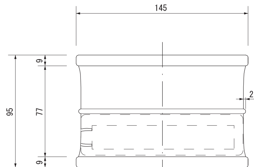
【上面図】
