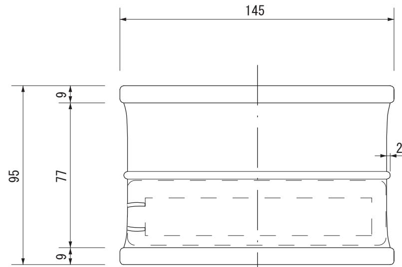
【上面図】
