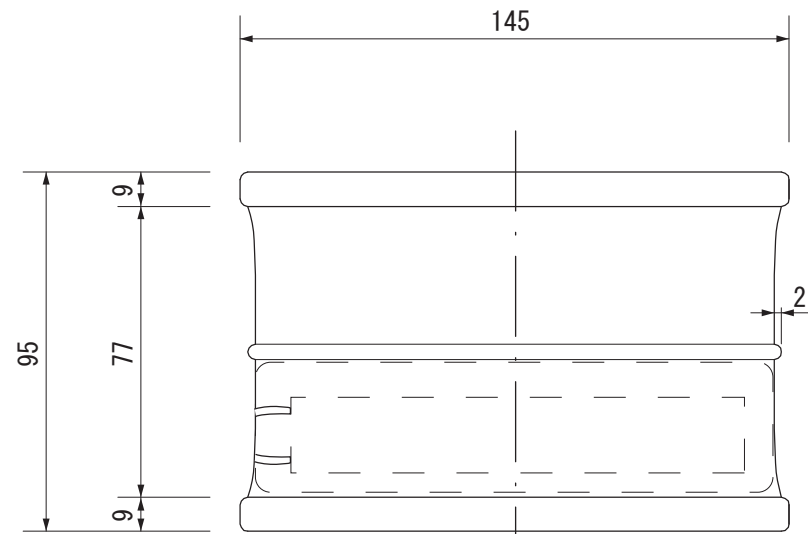
【上面図】
