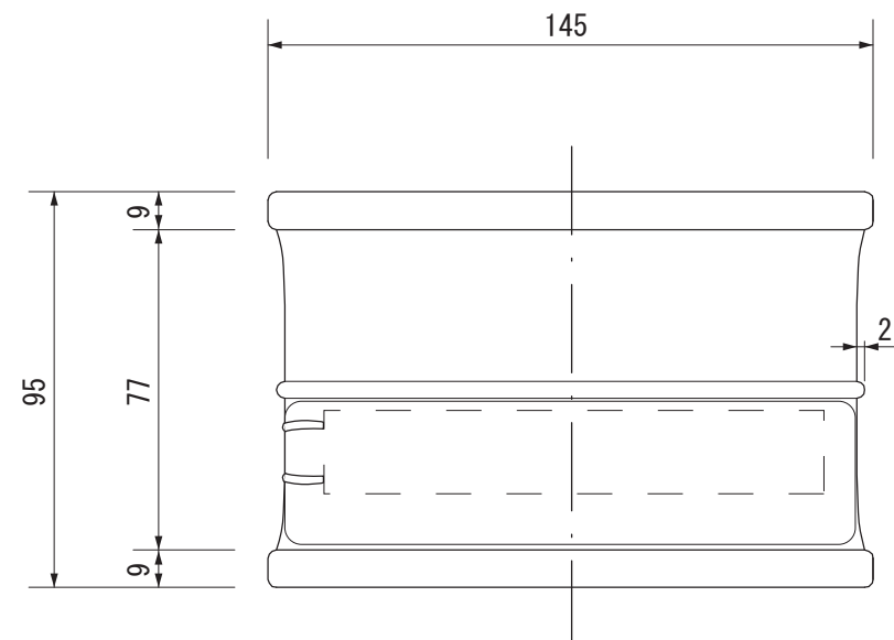
【上面図】
