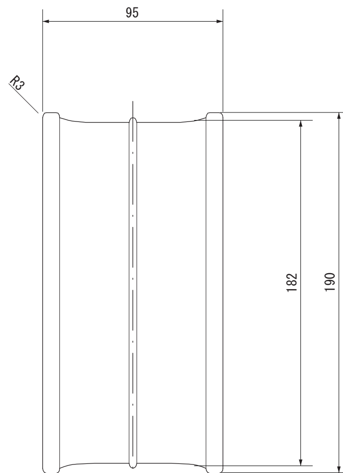
【側面図】
