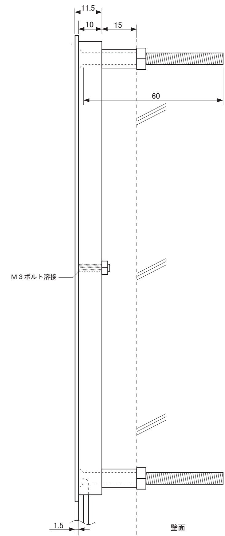
【側面図】
