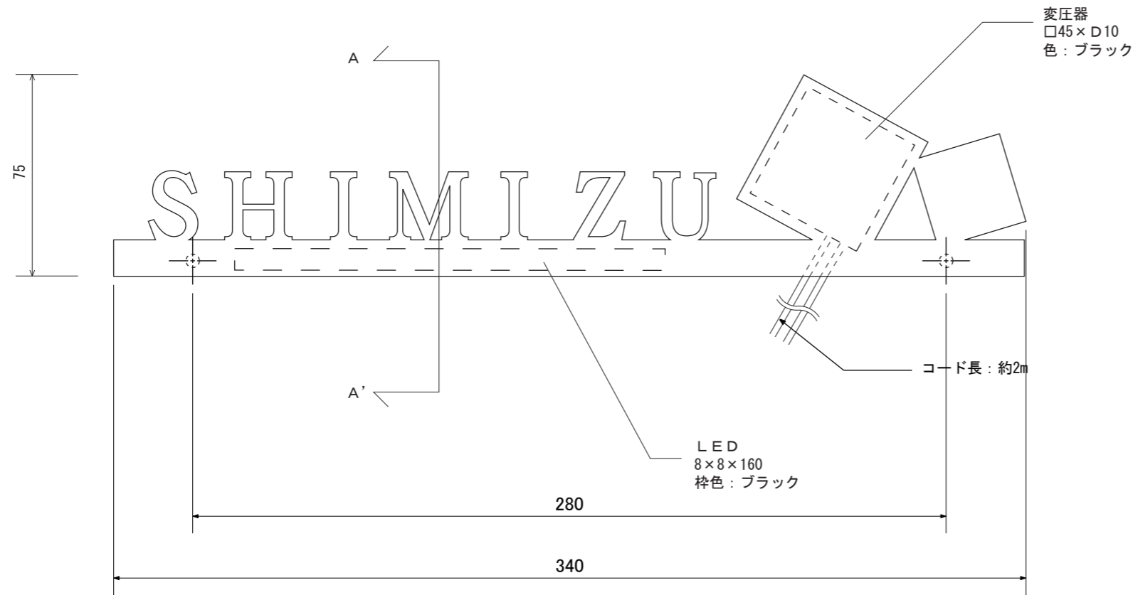
【正面図】
