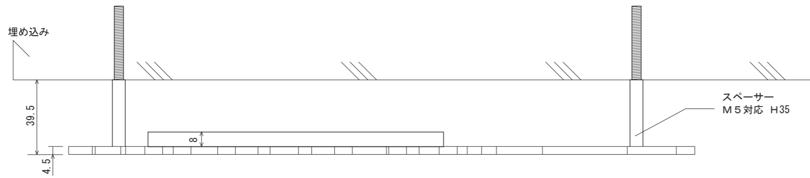
【上面図】
