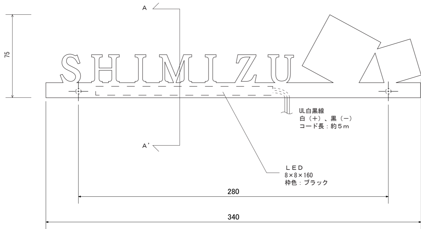
【正面図】
