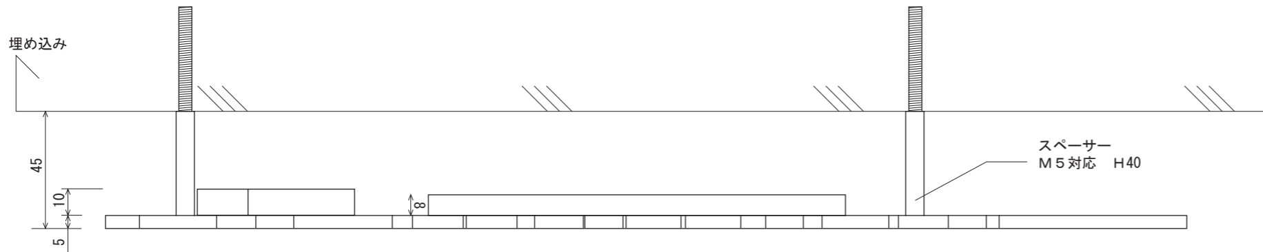
【上面図】
