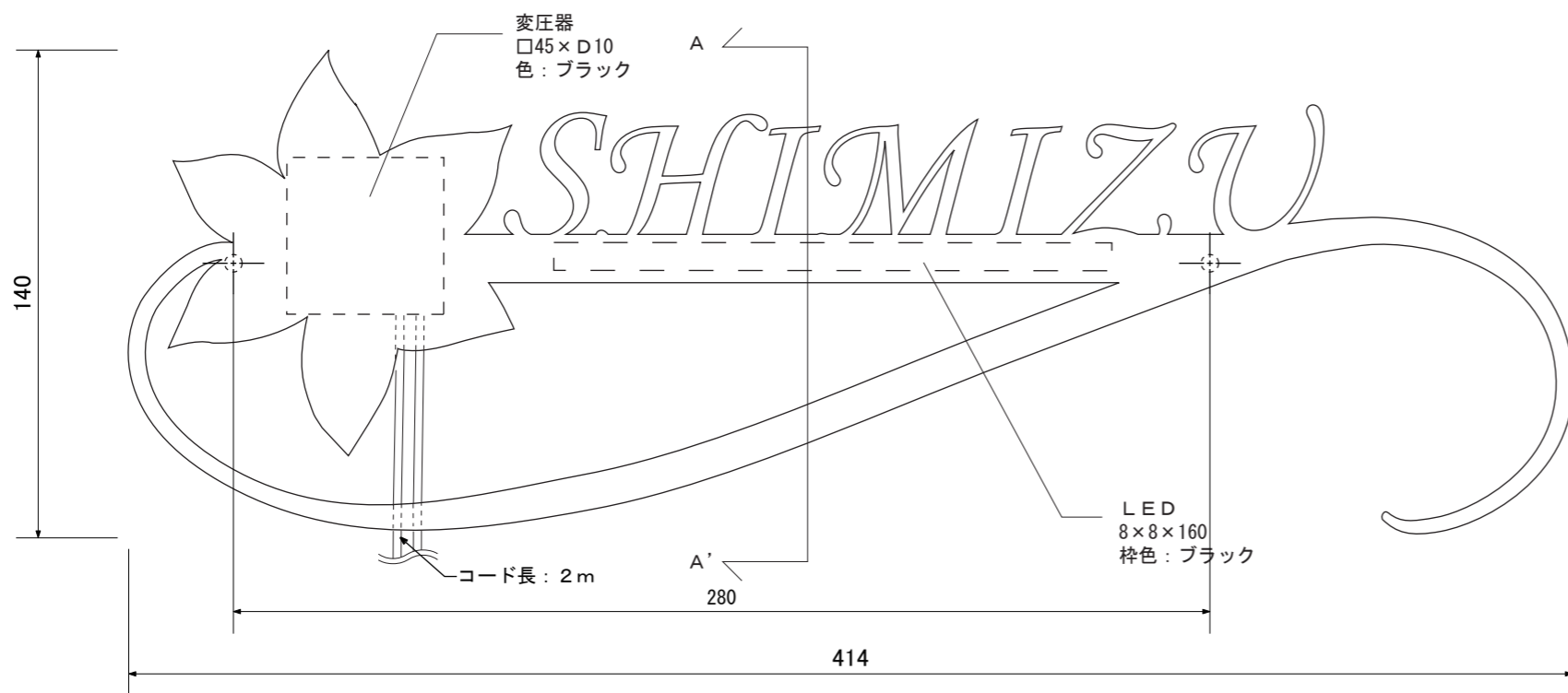
【正面図】
