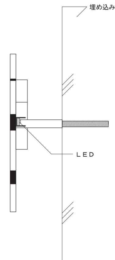
【A-A' 断面図】
