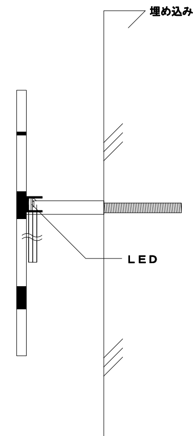
【A-A' 断面図】
