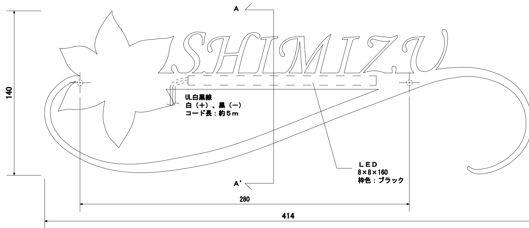
【正面図】
