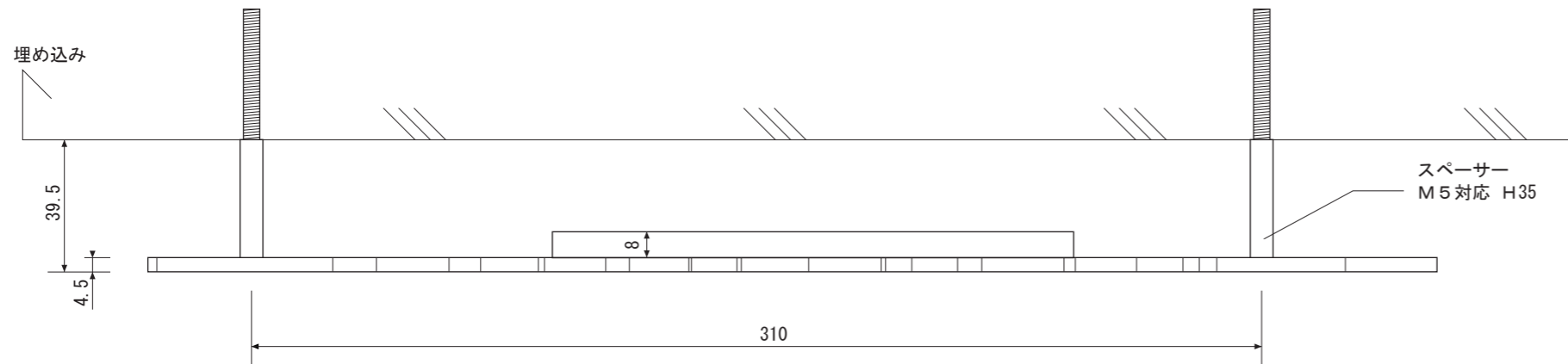
【上面図】
