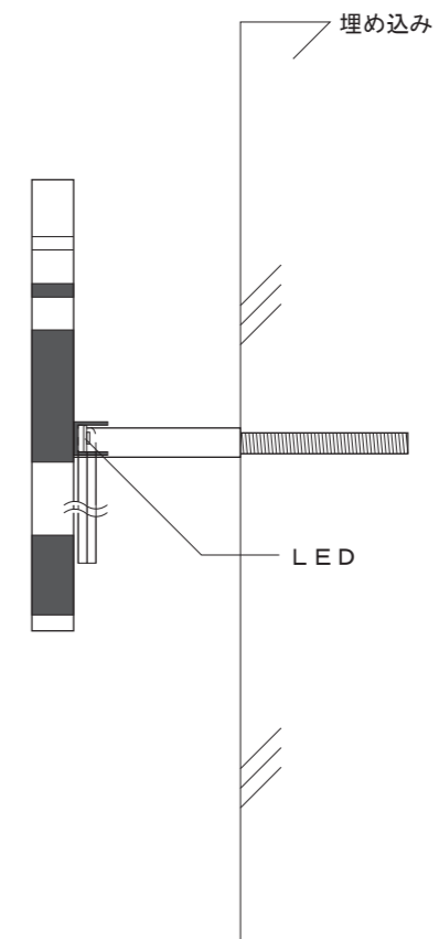
【A-A' 断面図】
