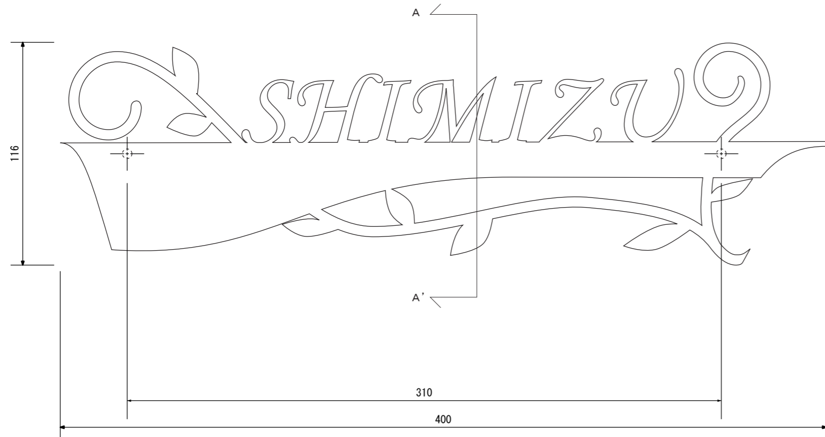
【正面図】
