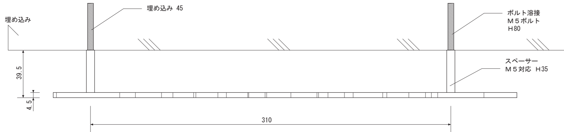
【上面図】
