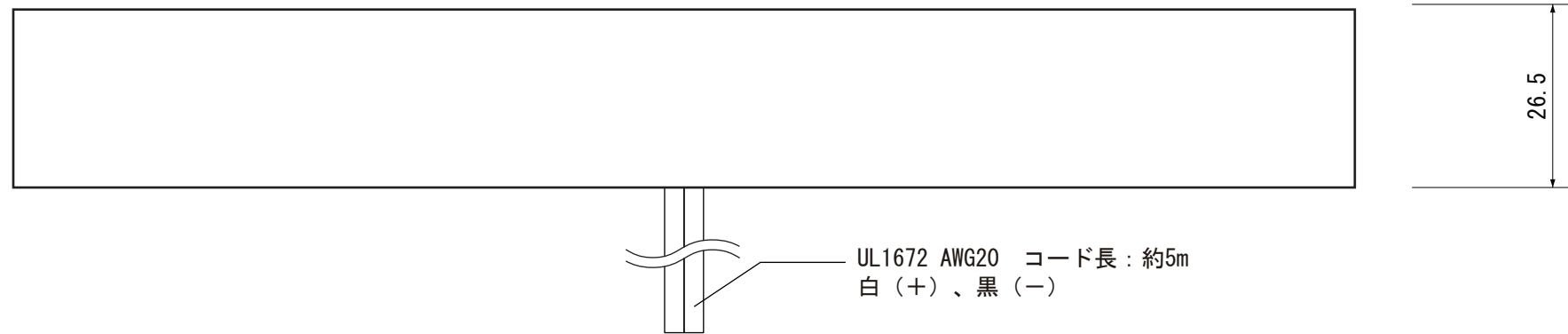
【側面図】
