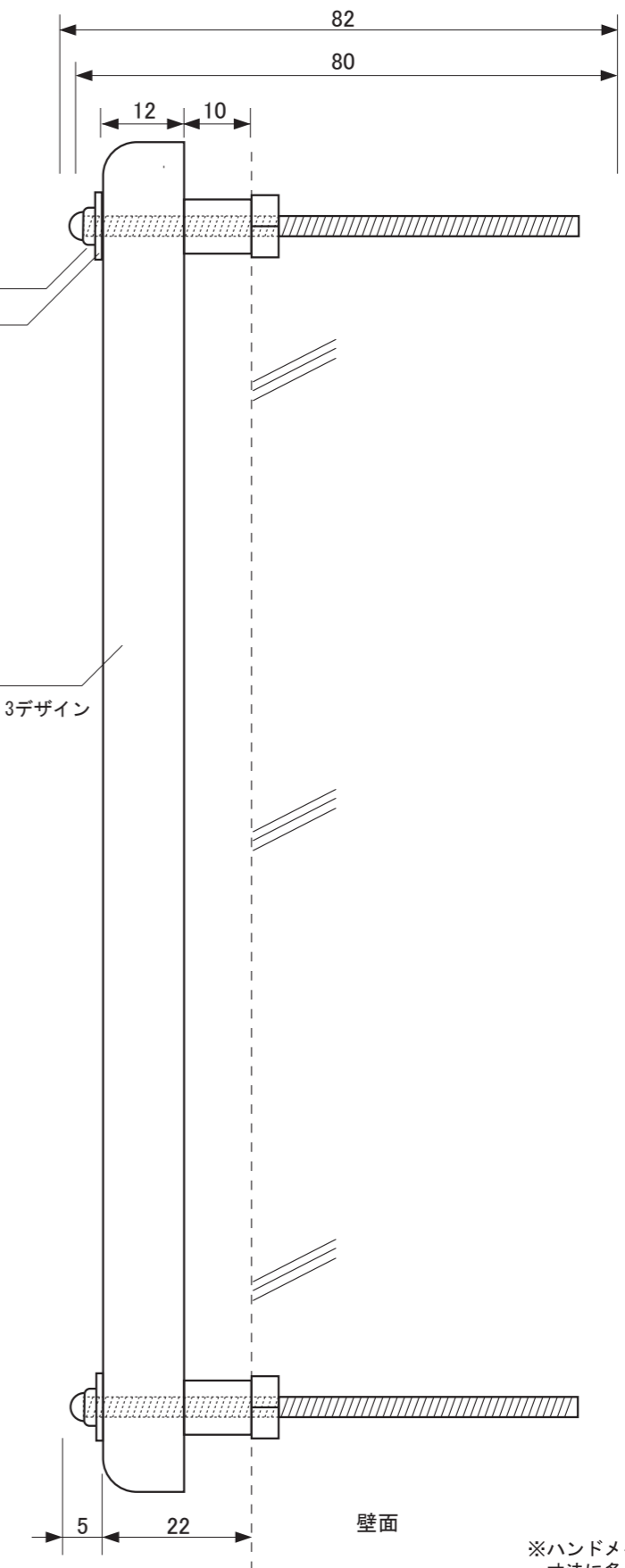
【側面図】
