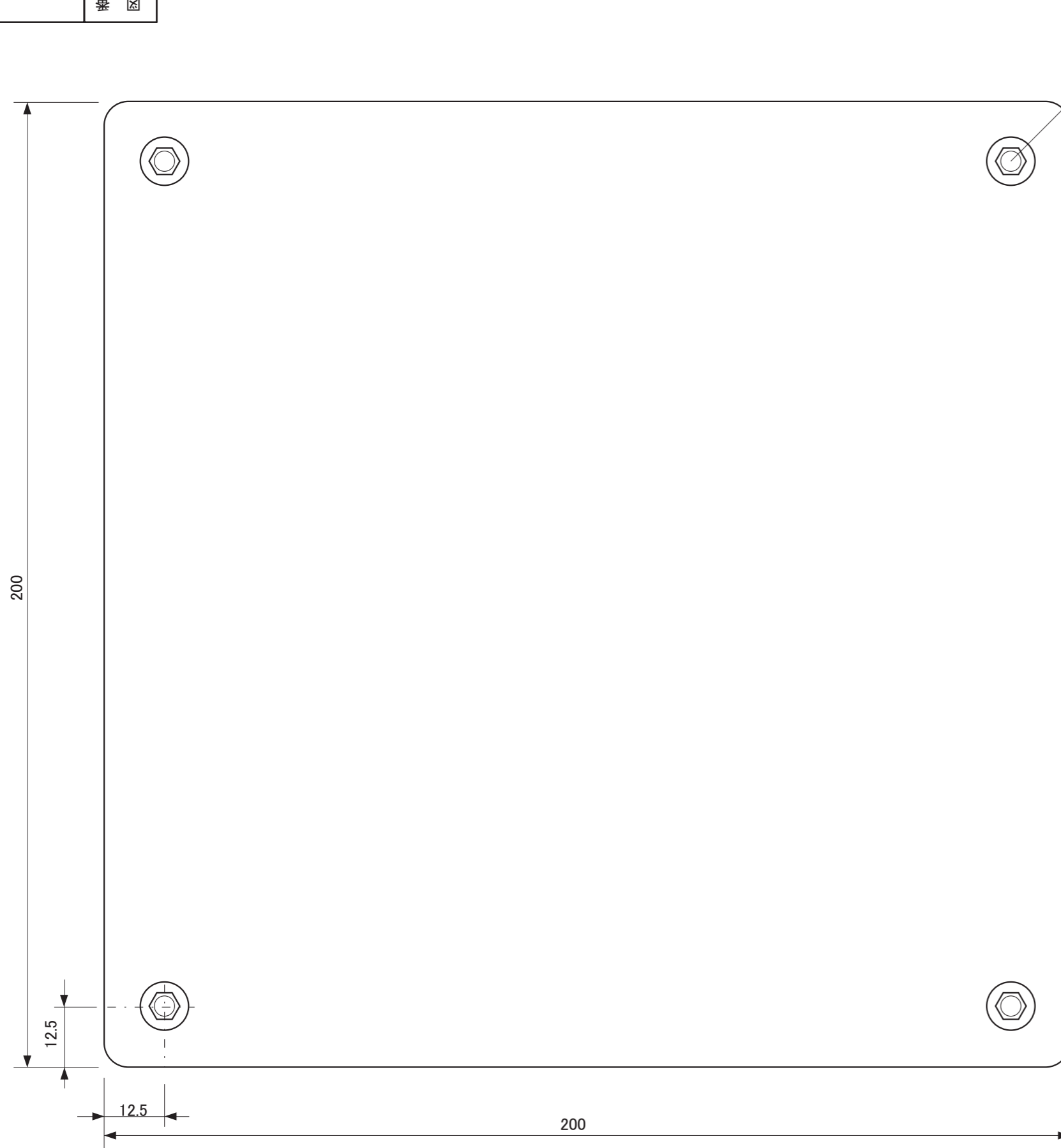
【正面図】
