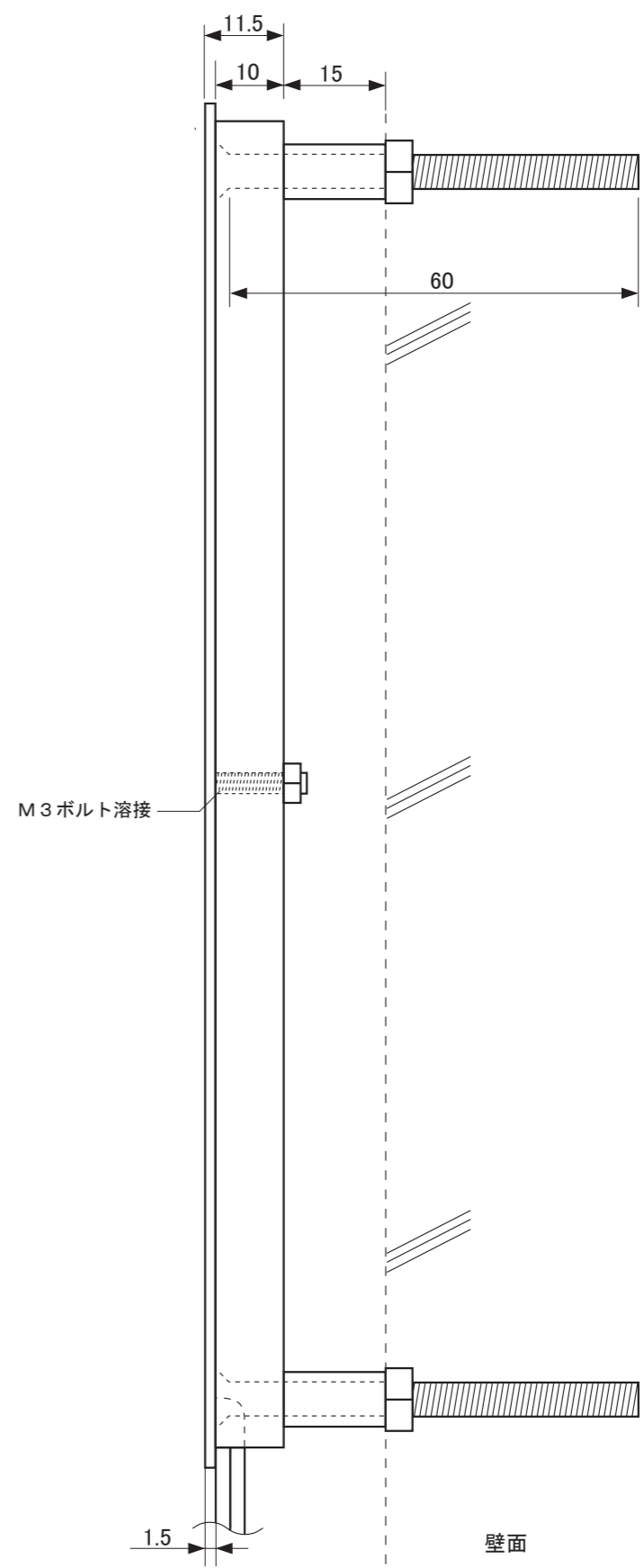
【側面図】
