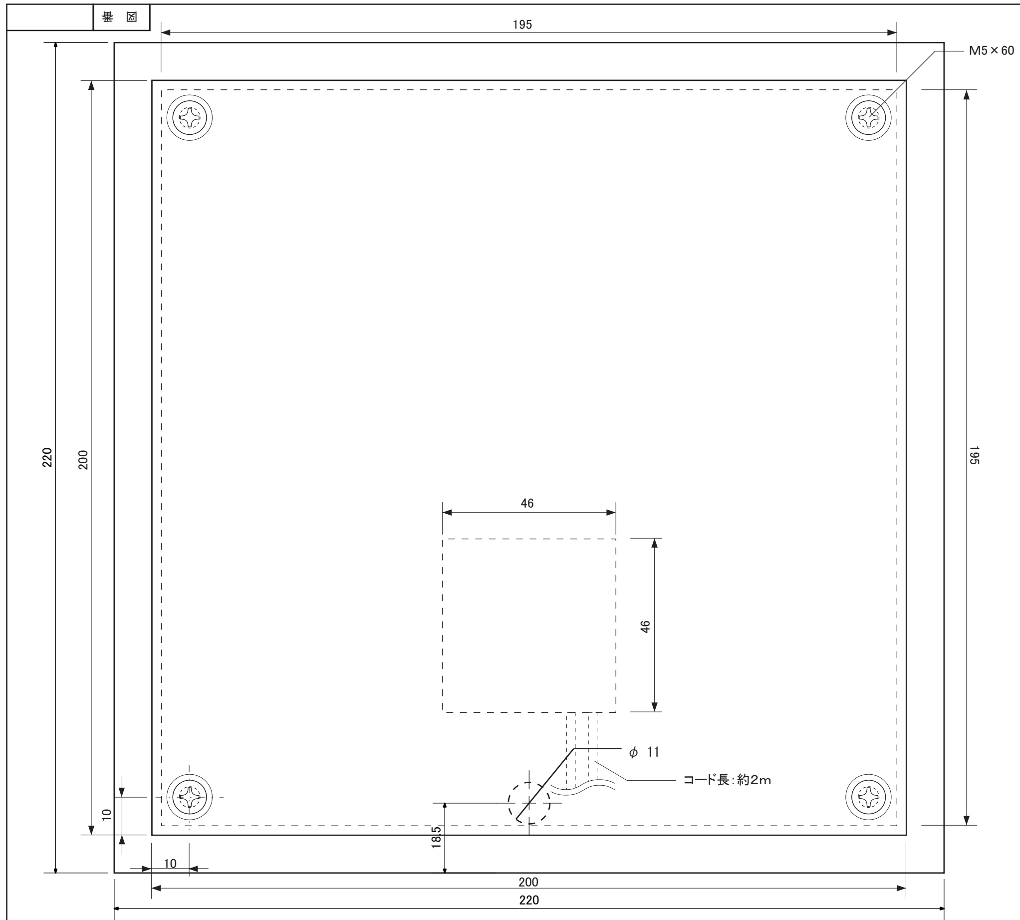
【正面図】
