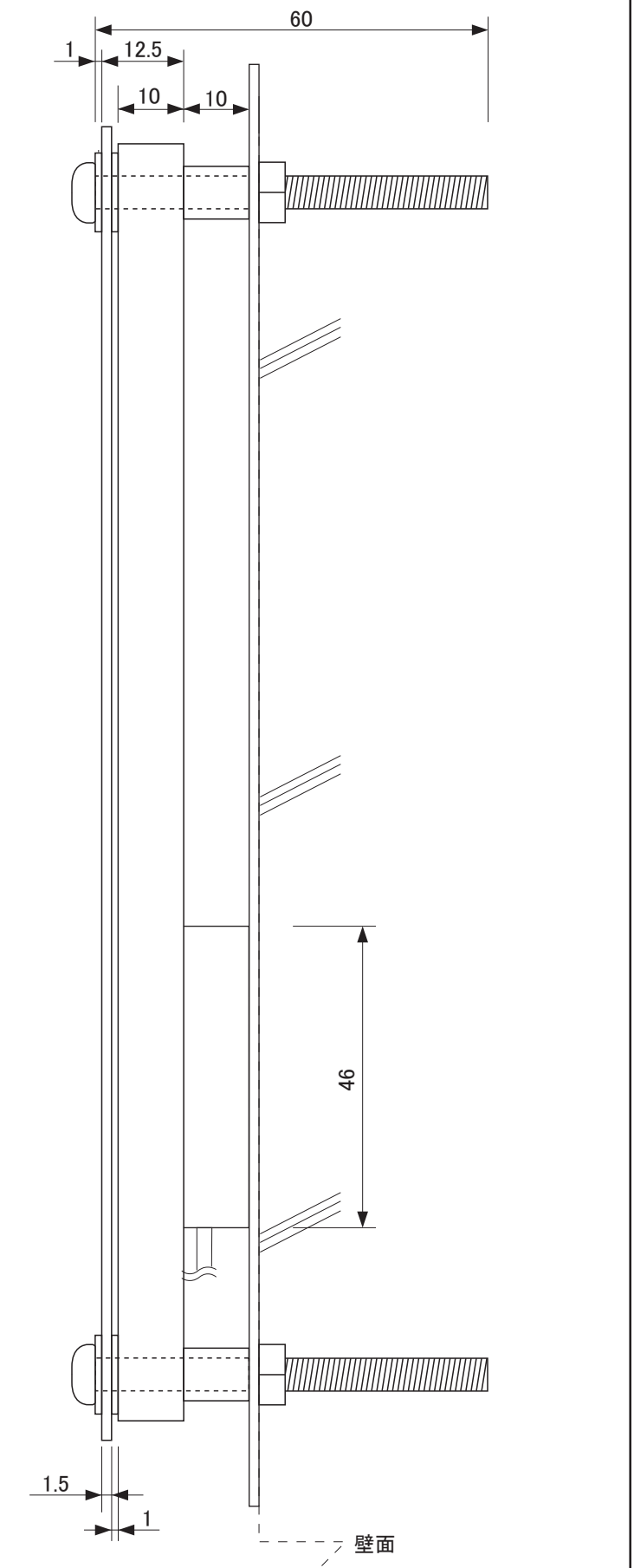
【側面図】
