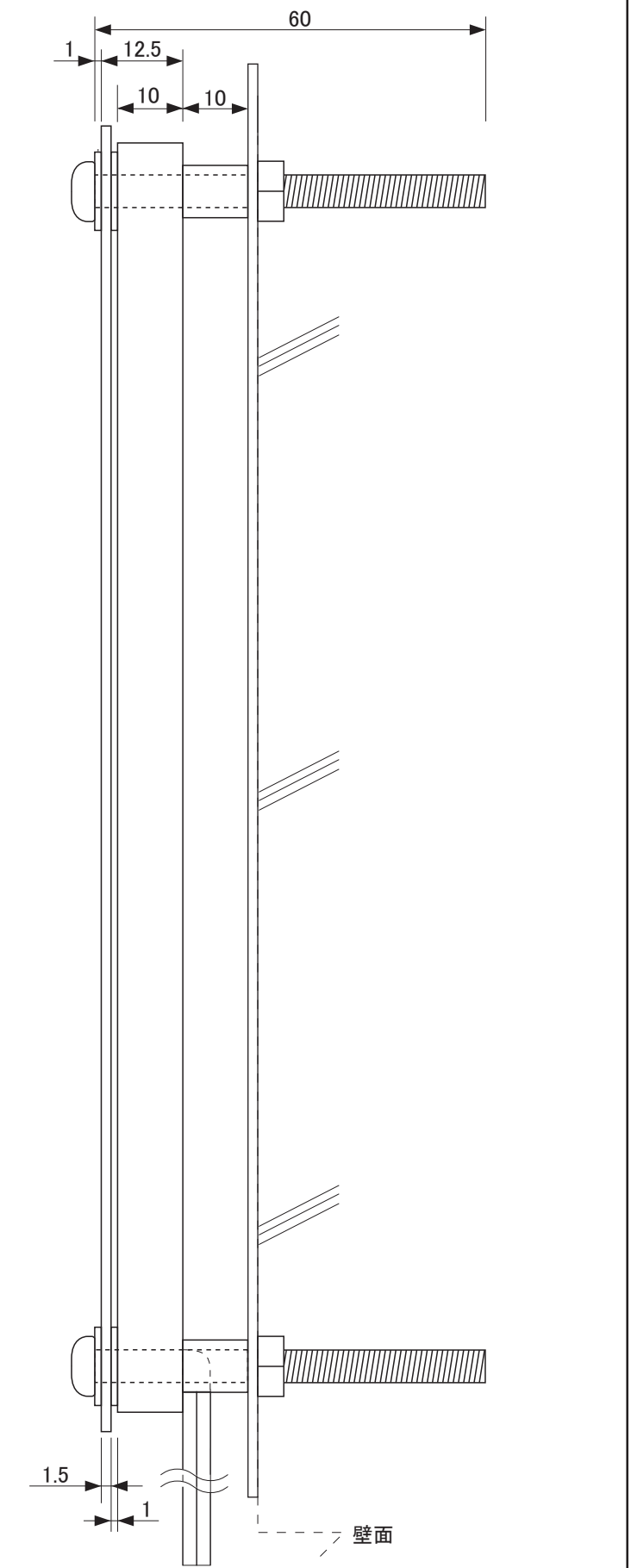
【側面図】
