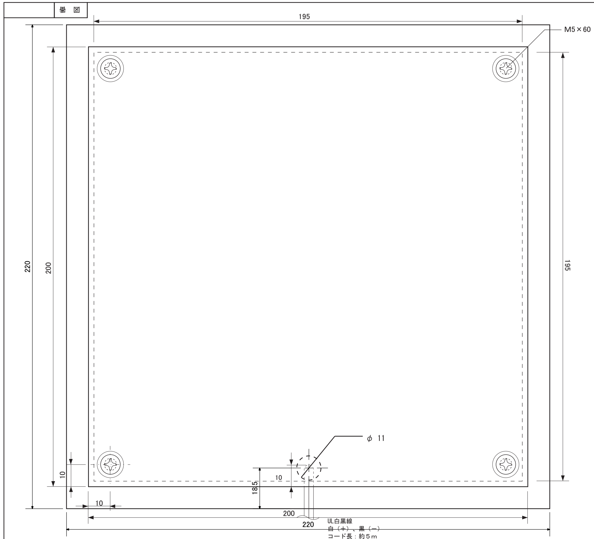
【正面図】
