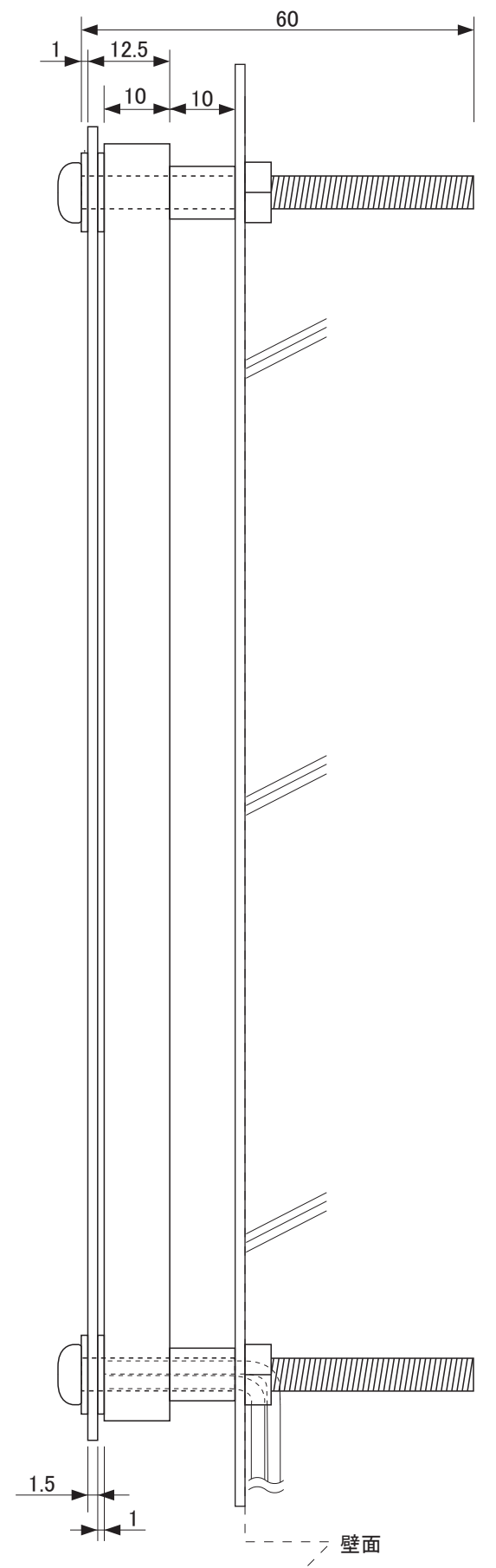
【側面図】
