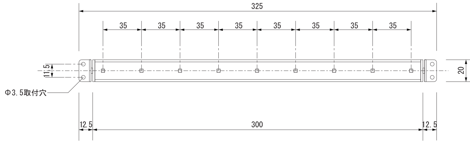
【上面図】
