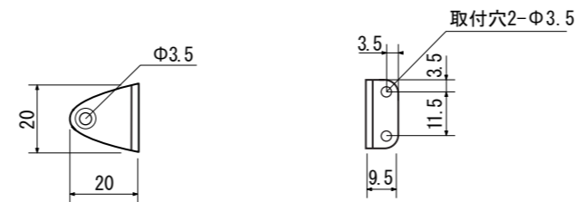
【側面図】
