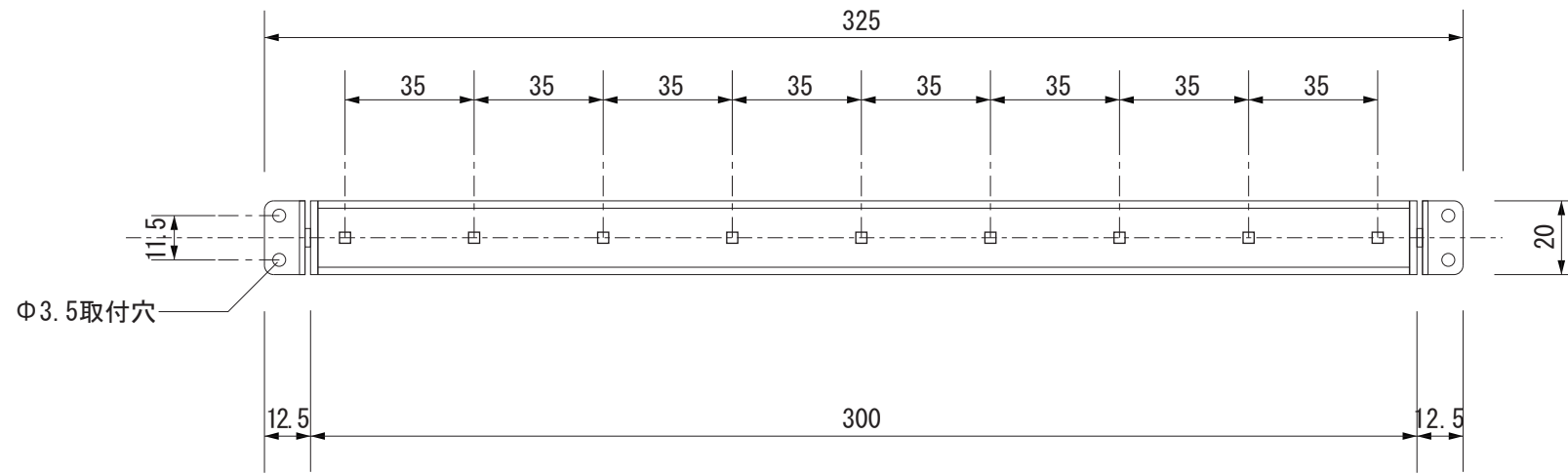
【上面図】
