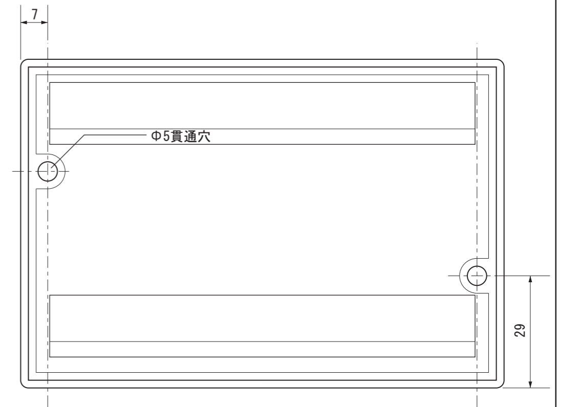
【背面図】
