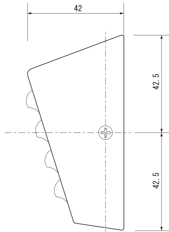
【側面図】
