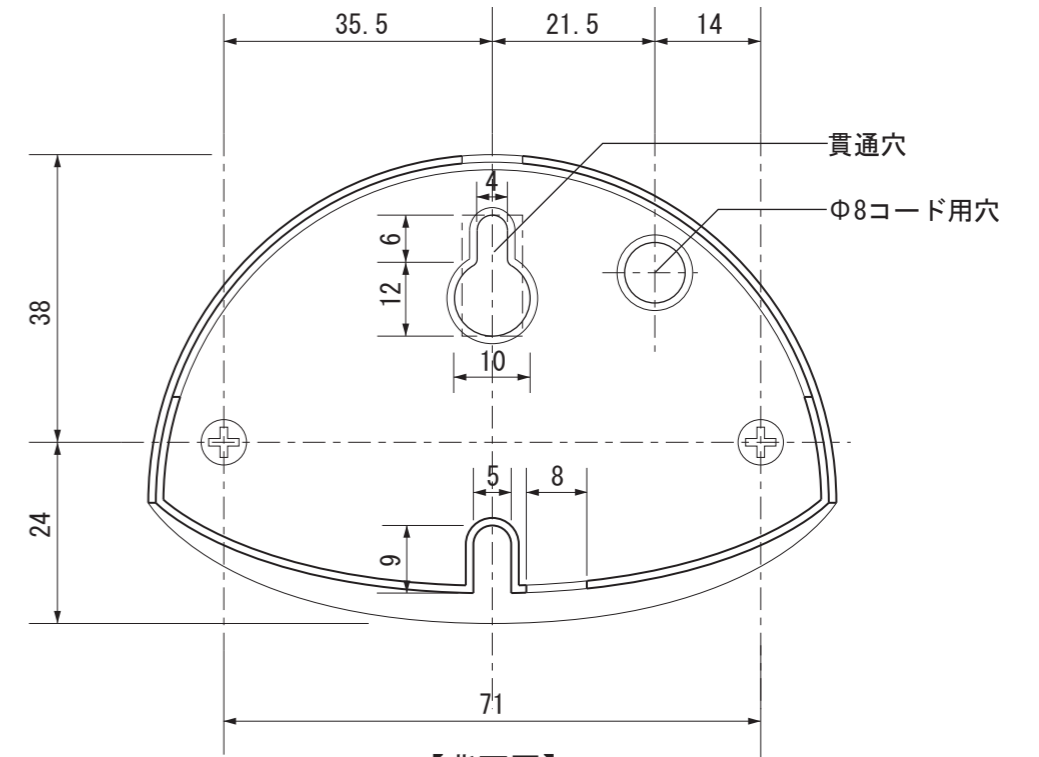
【背面図】
