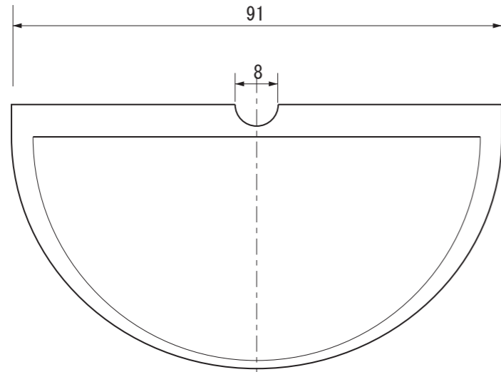
【上面図】
