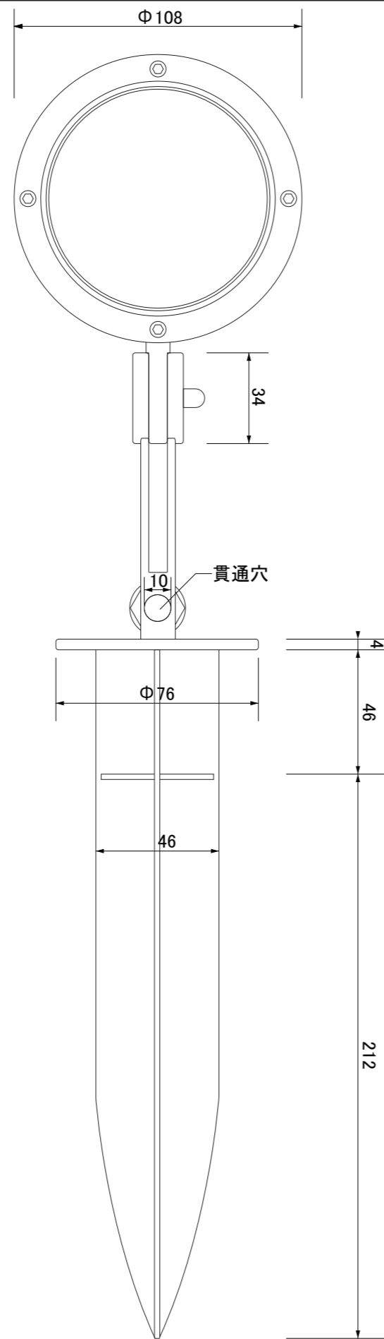
【正面図】
