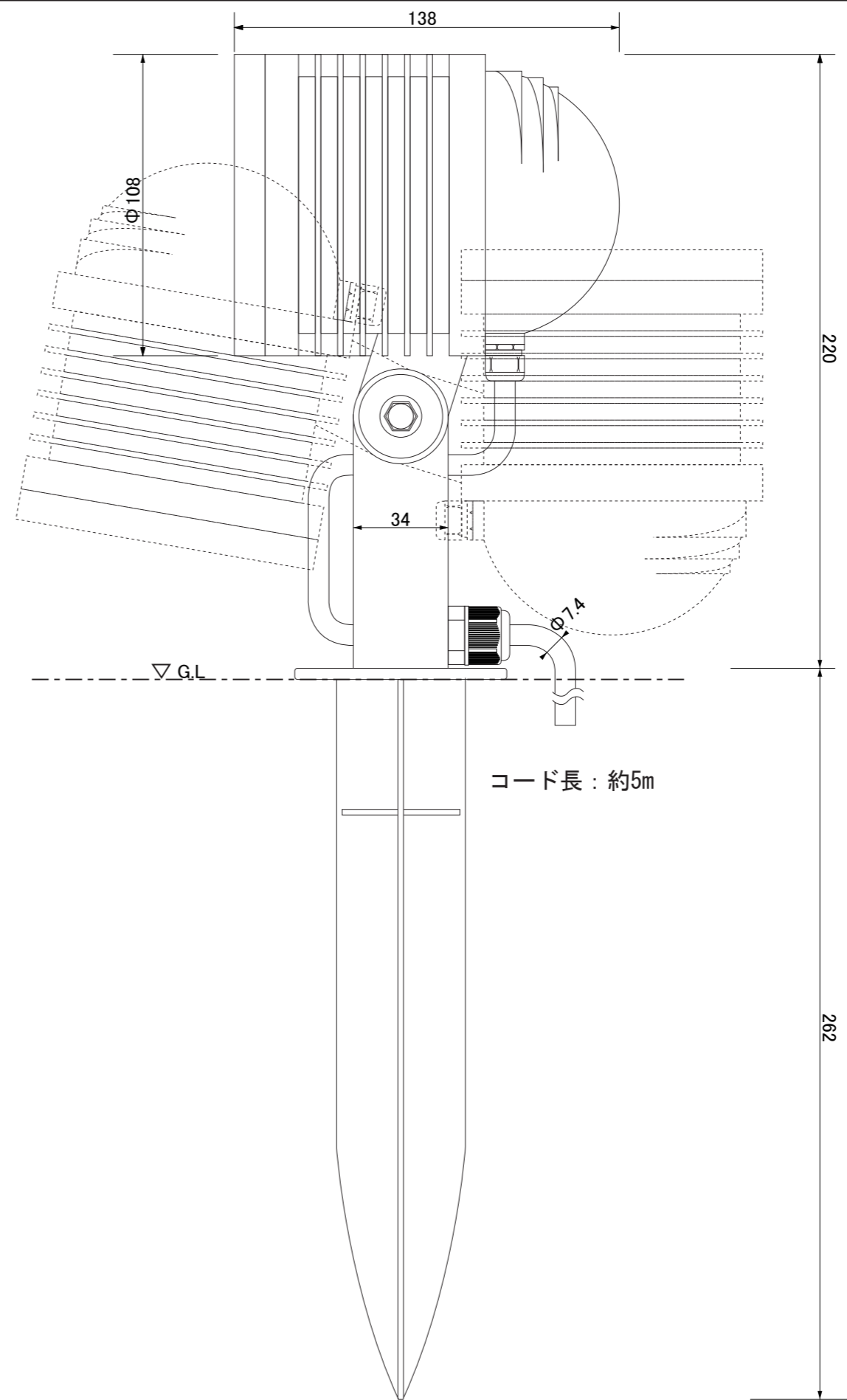
【正面図】
