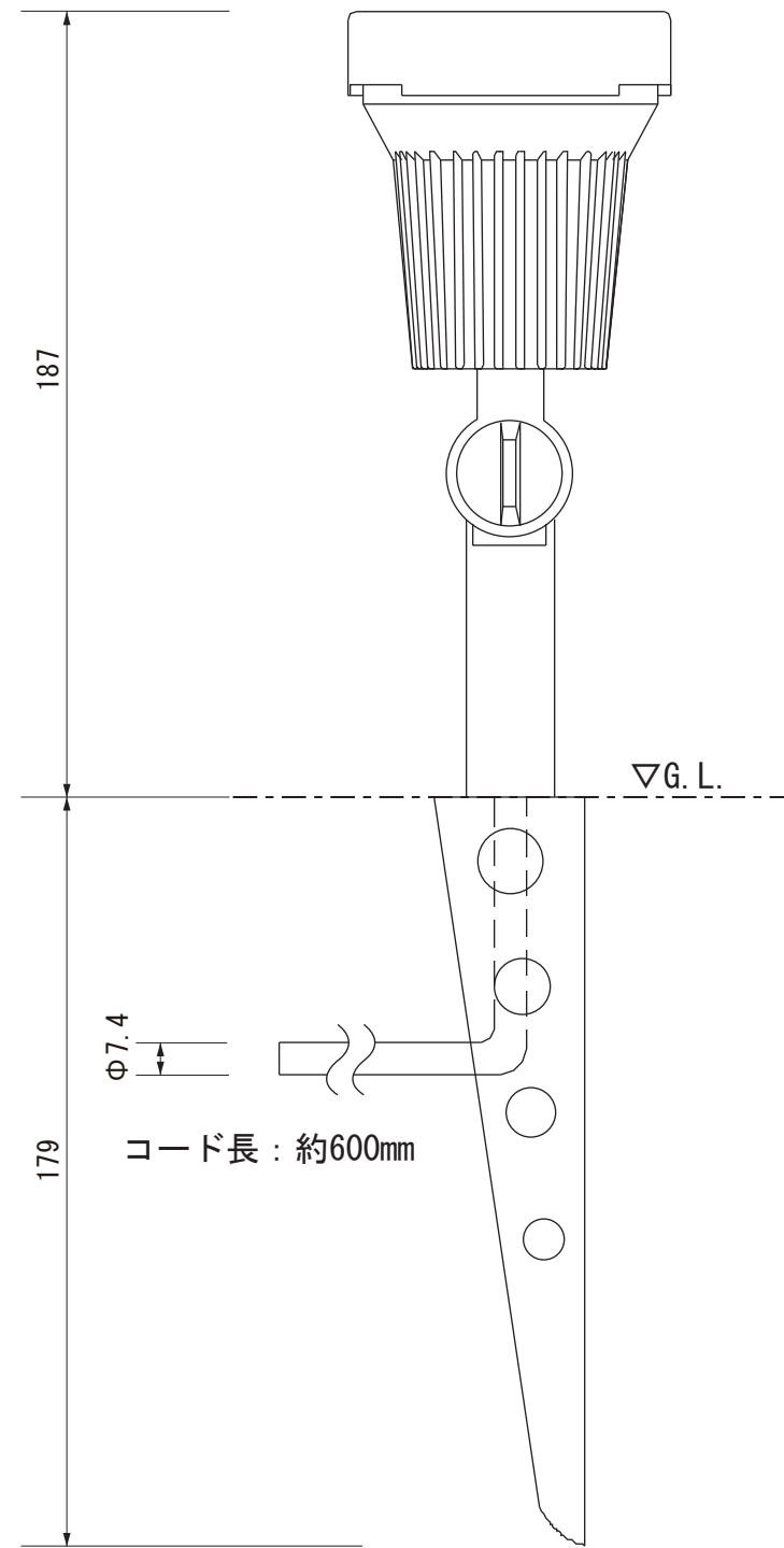
【正面図】
