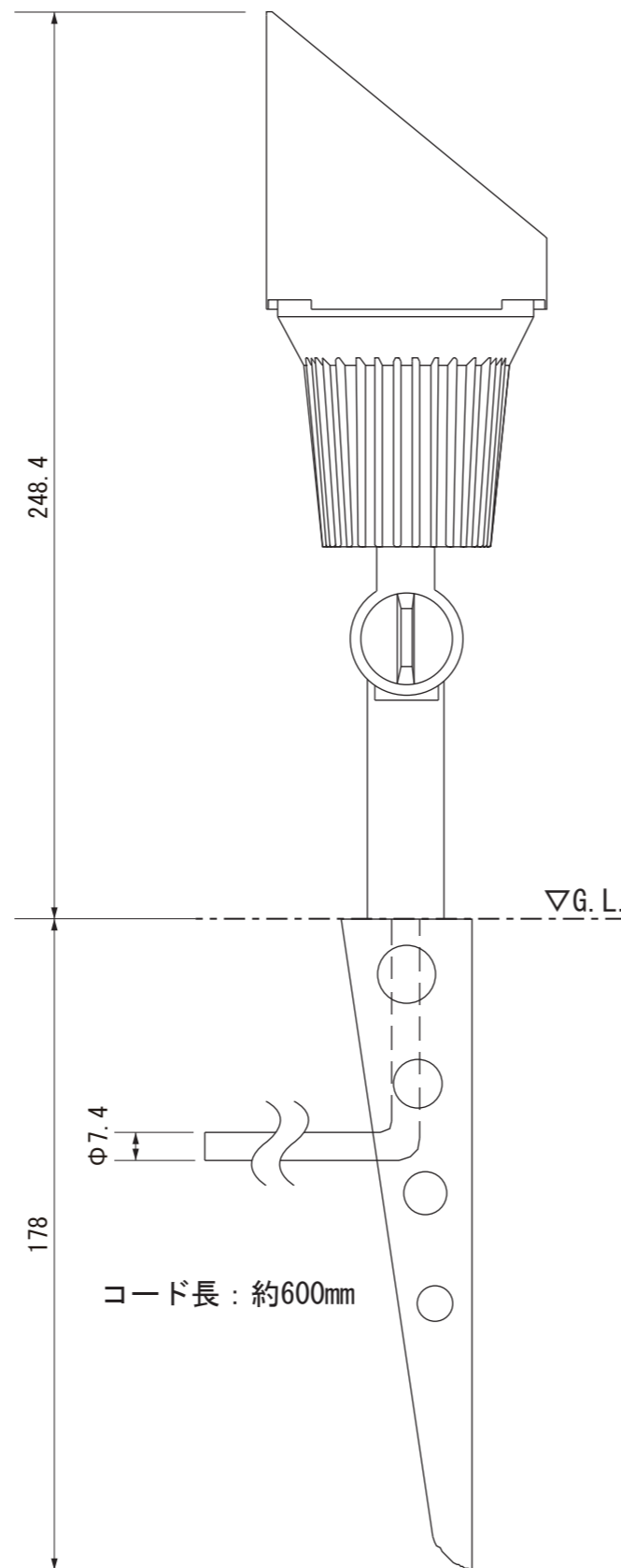
【正面図】
