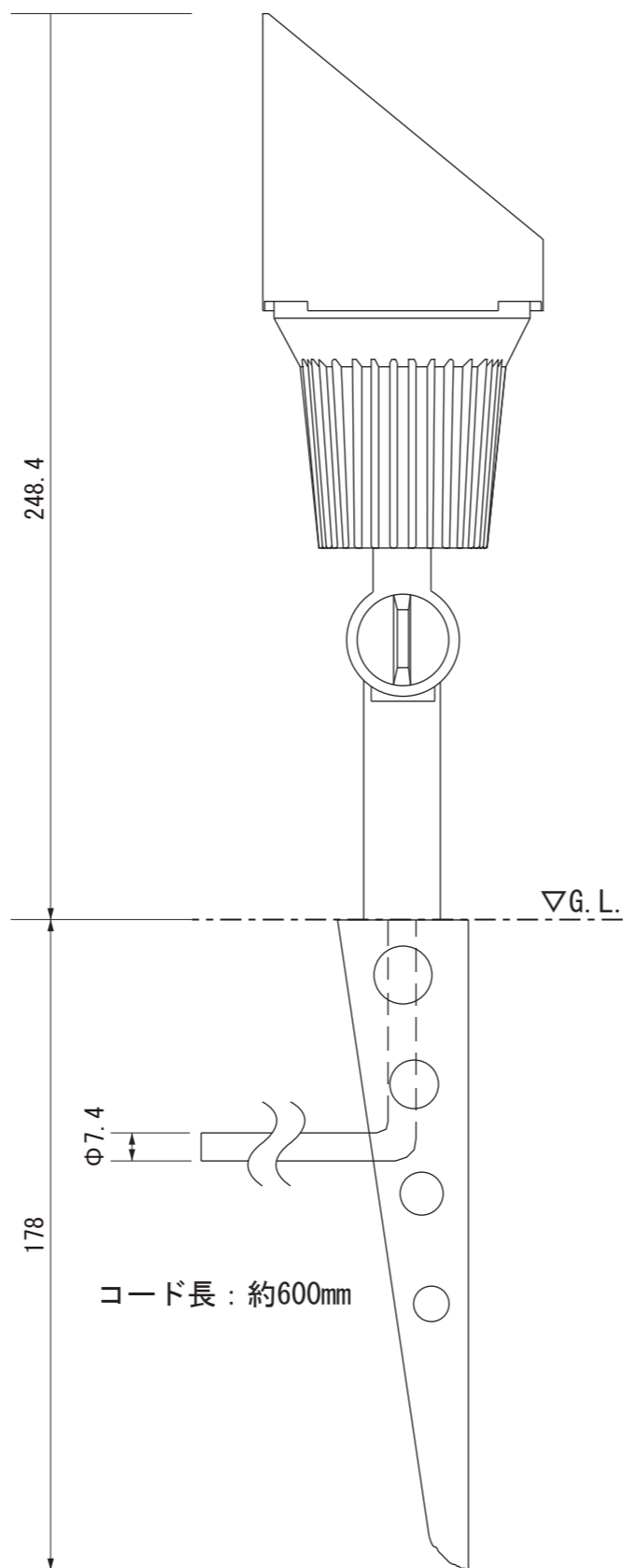
【正面図】
