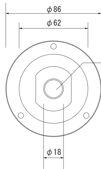
【底面図】
