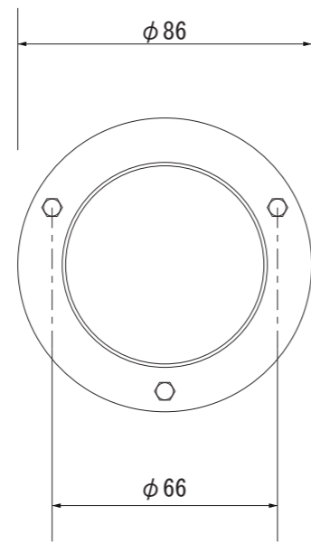
【上面図】
