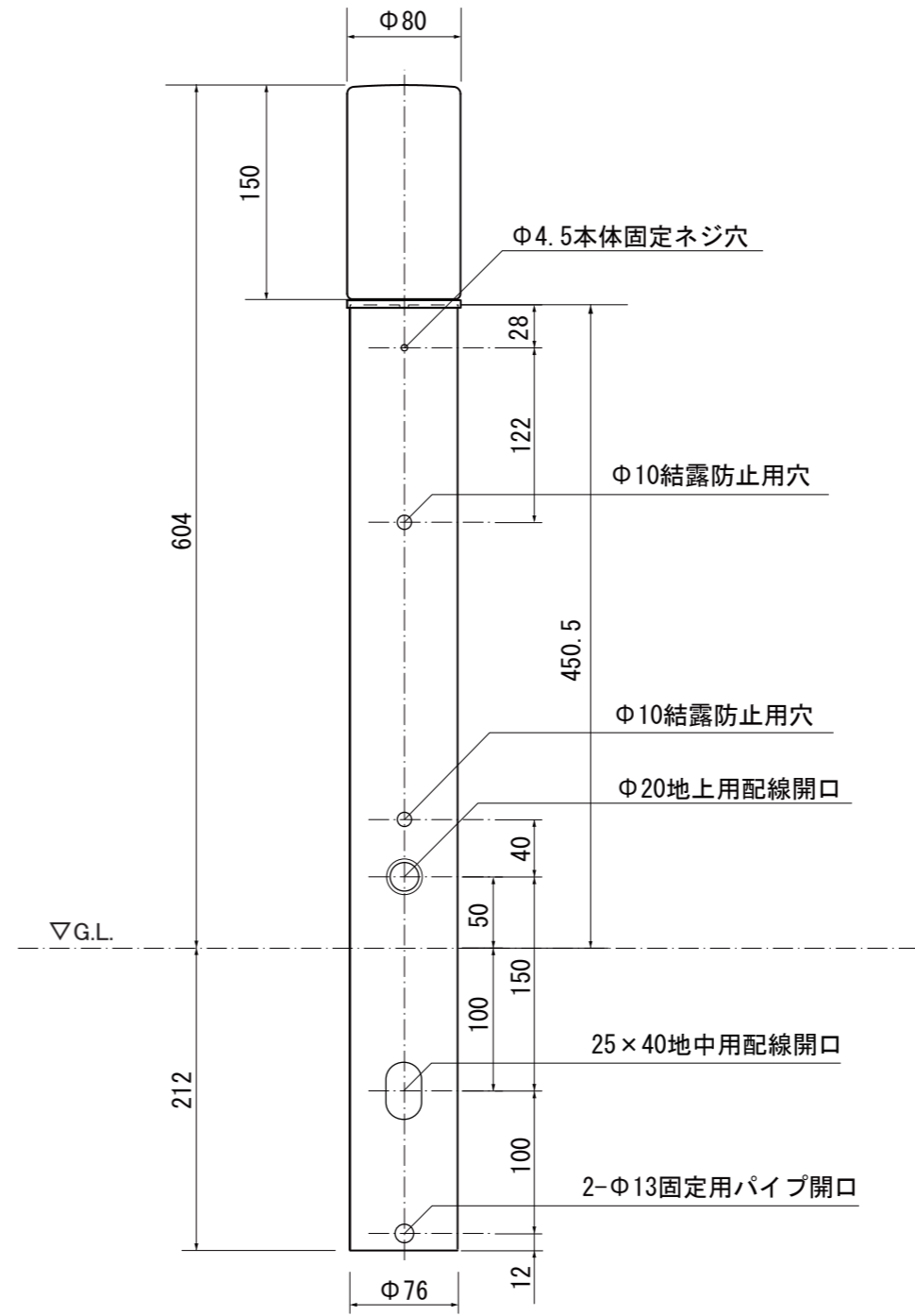
【正面図】
