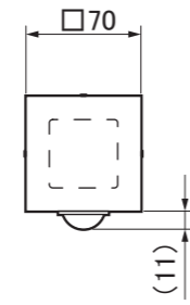
【上面図】
