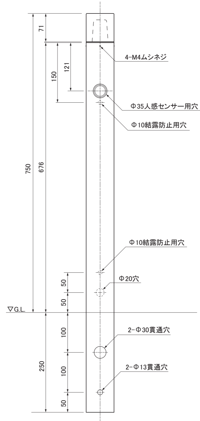
【正面図】
