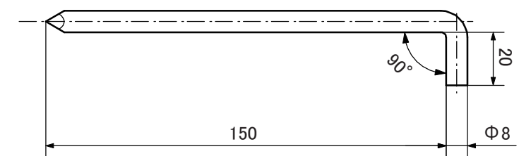
【付属ペグ】
