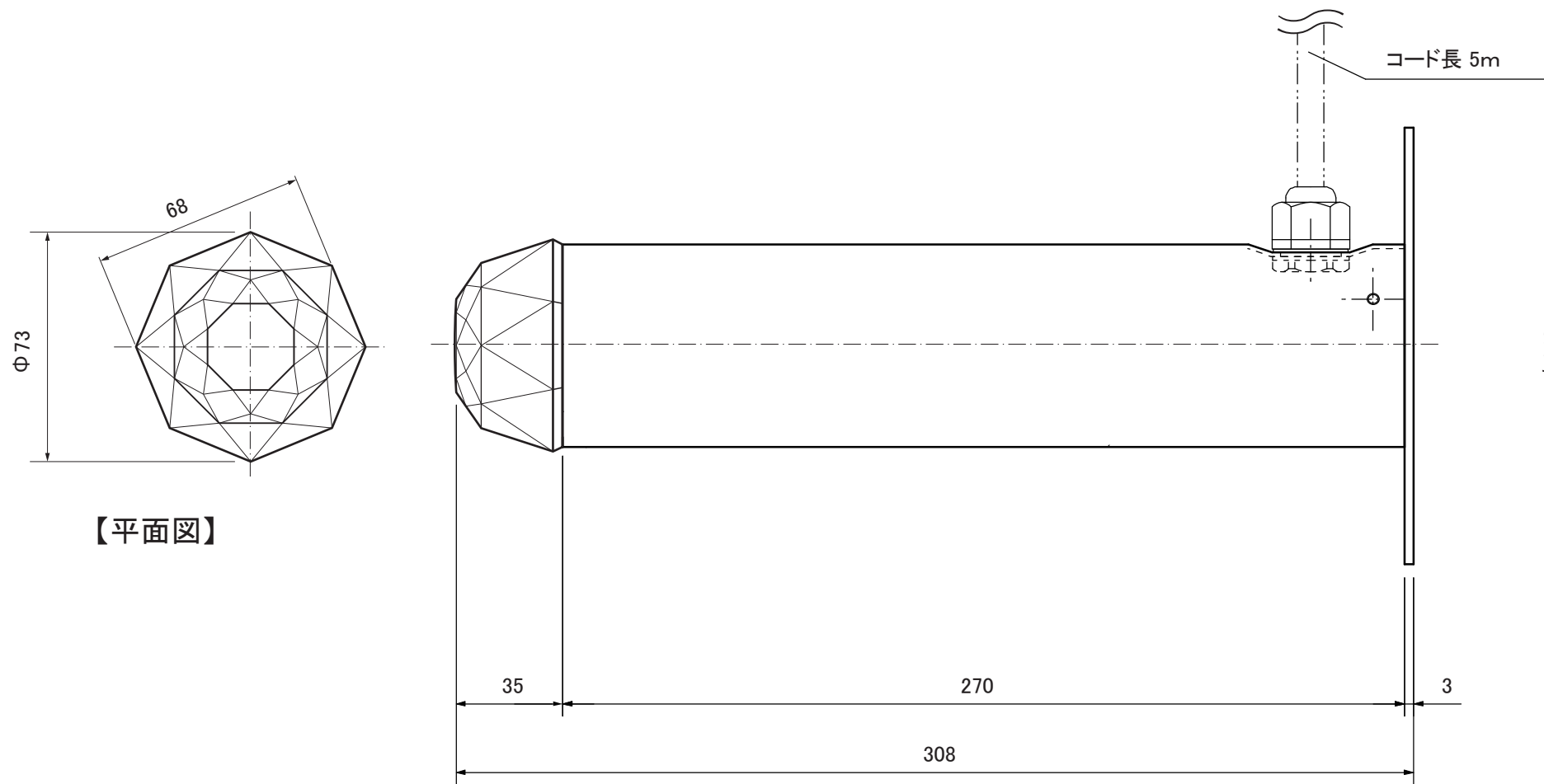
【正面図】
