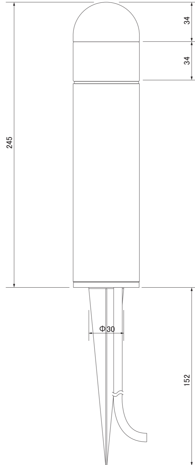
【正面図】
