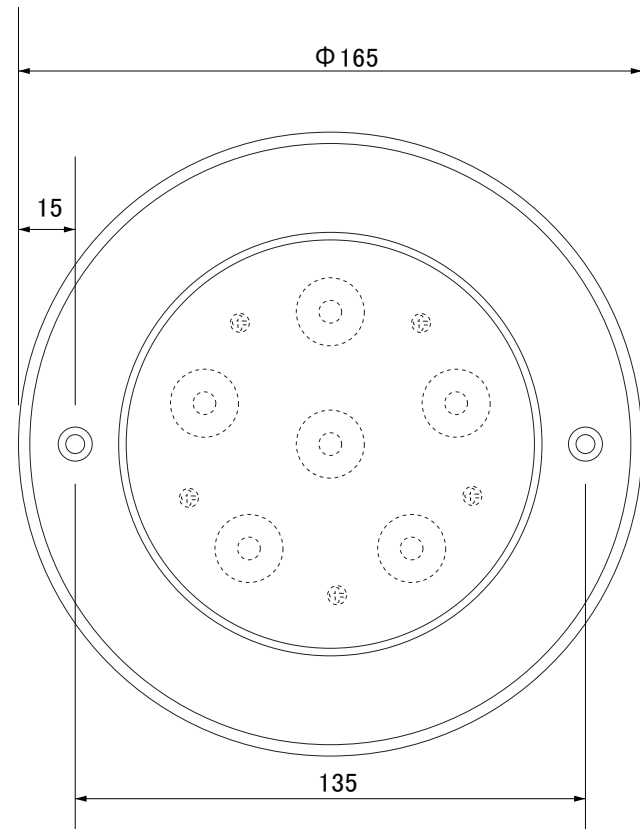
【正面図】
