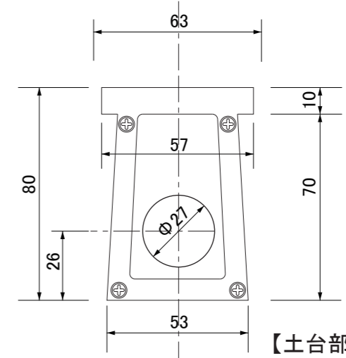
【土台部正面図】
