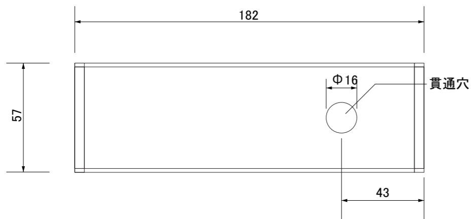
【土台部底面図】
