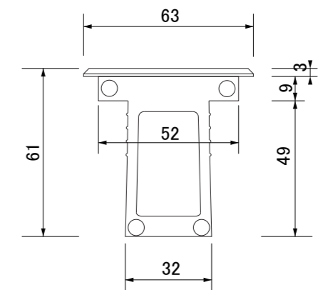
【本体側面図】
