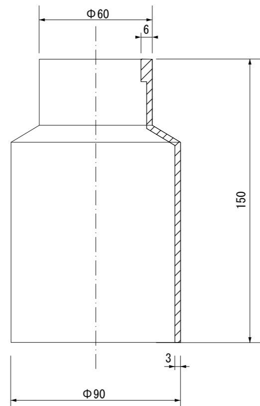
【土台部 正面図】
