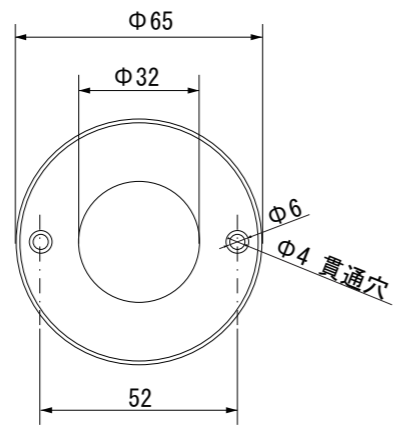
【上面図】
