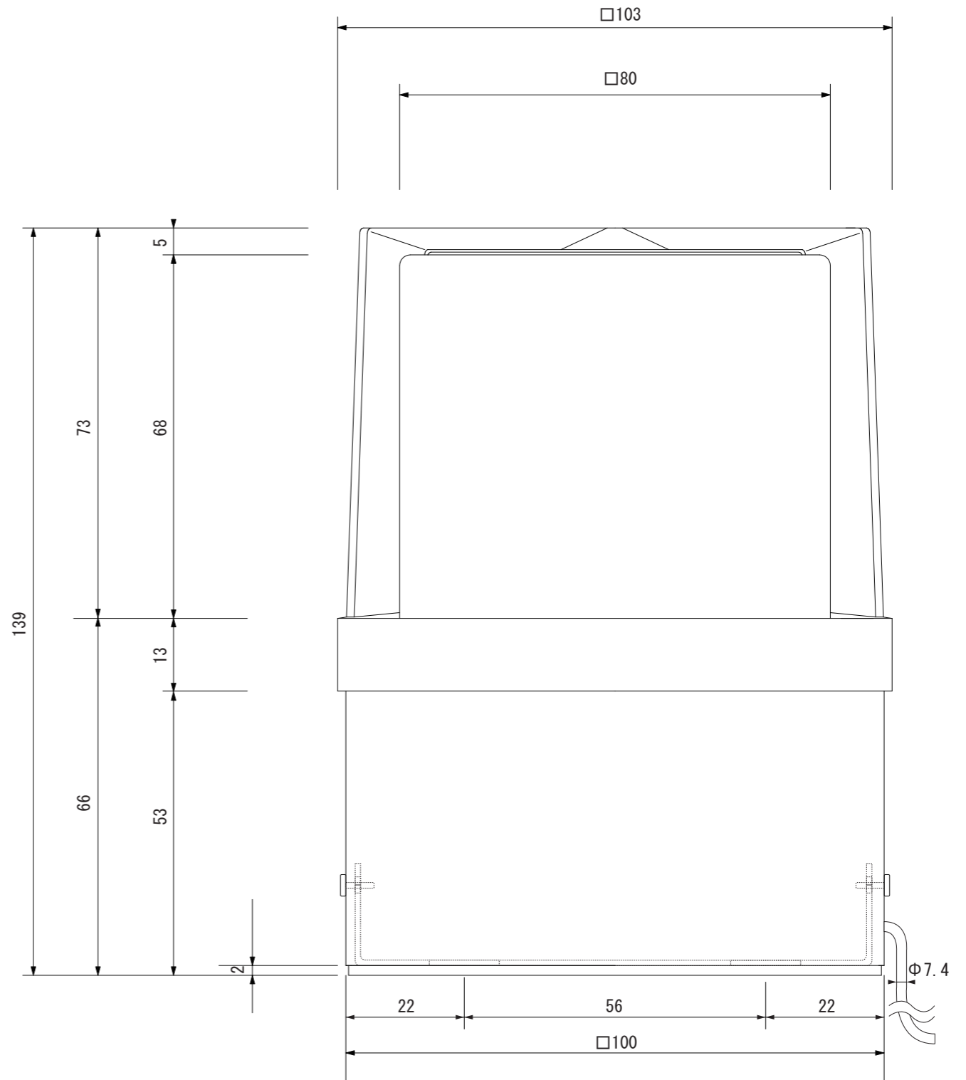
【正面図】
