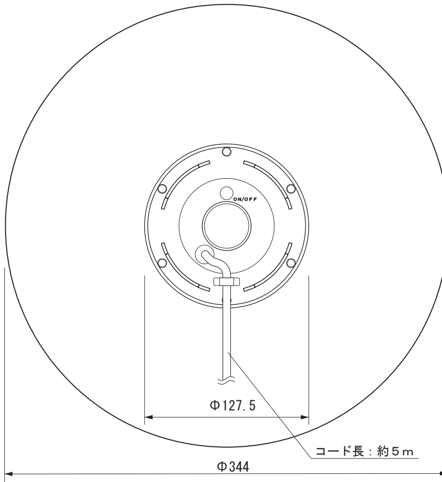
【底面図】
