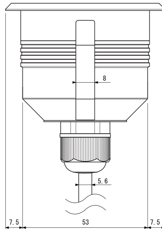
【側面図】
