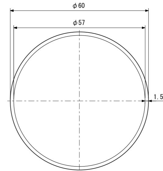
【土台部上面図】
