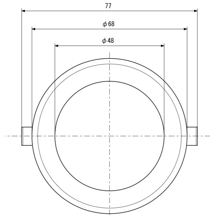
【上面図】
