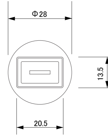
【底面図】
