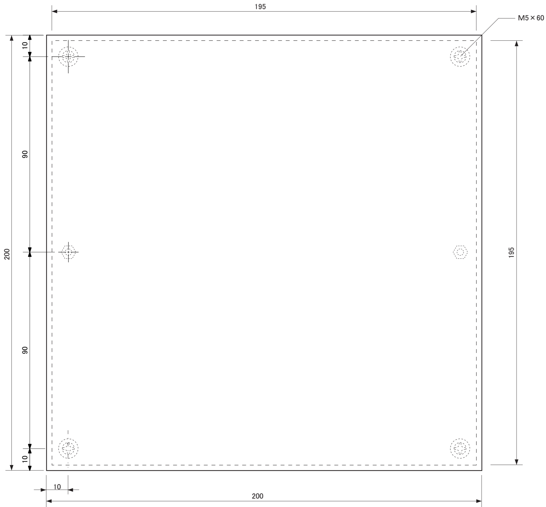
【正面図】
