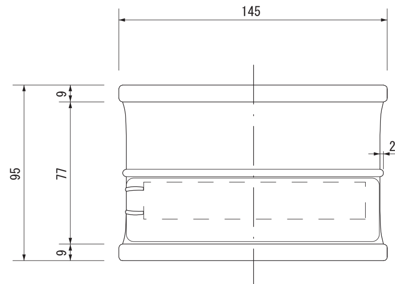
【上面図】
