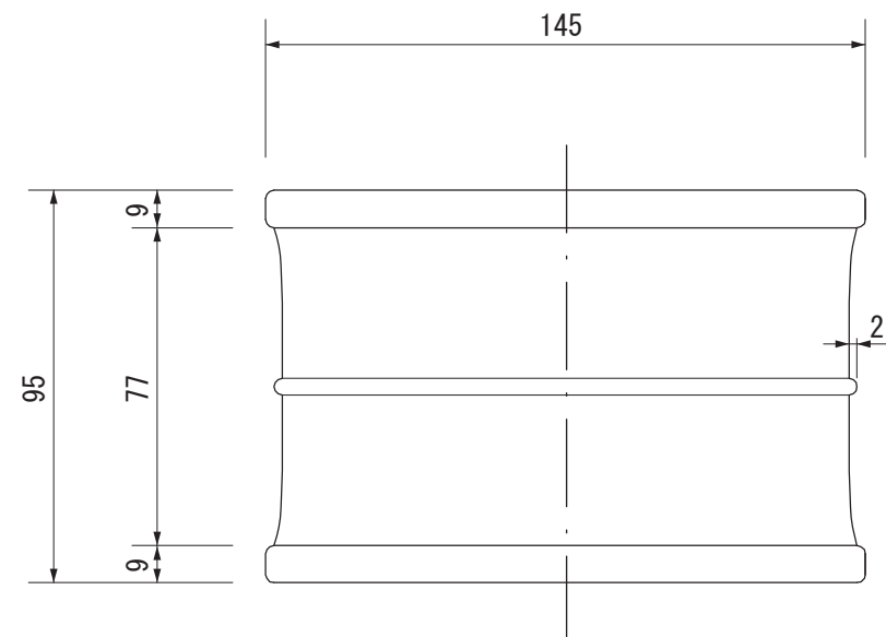
【上面図】
